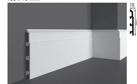
HCR 510 (F) 150 x 18 mm
