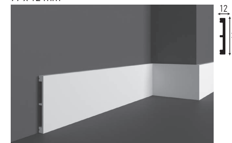
HCR 520 (F) 99 x 12 mm
