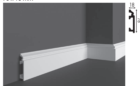
HCR 507 (F) 78 x 18 mm
