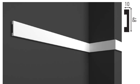
HCR 504 (F) 48 x 10 mm
