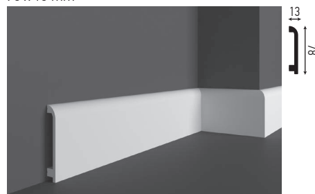
HCR 519 (F) 78 x 13 mm
